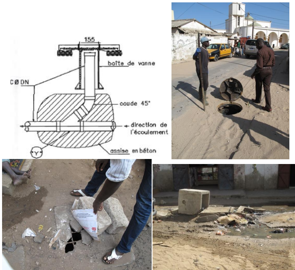
A gauche : cheminée de visite (source : ONAS). Au centre : couvercle de regard en fonte sur un réseau ONAS à Yoff (Dakar). A droite : couvercle en béton abîmé à Baraka (Dakar) et regard bouché par les déchets à Rufisque (sur la voie, renversé, l'ancien regard déposé).
